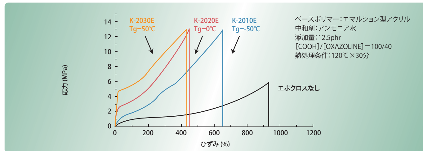
フィルム引張り強度試験結果
