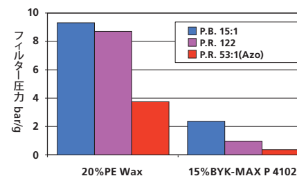
事例1. 有機顔料40%添加LDPE フィルター圧力 (ISO 23900-5) 低減
